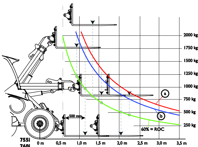
Diagramme de charge 755i / 760i
